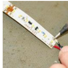
Beste Verbindung durch Kabelanlötlung an vorverzinnnten Lötspots.
